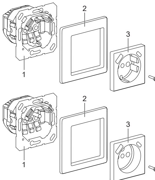
Afb. 1: Constructie apparaat
