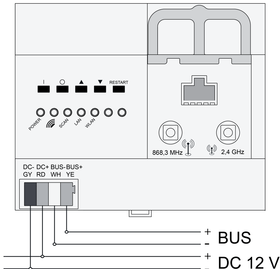
Afbeelding 4: Aansluiting van de voedingsspanning REG
