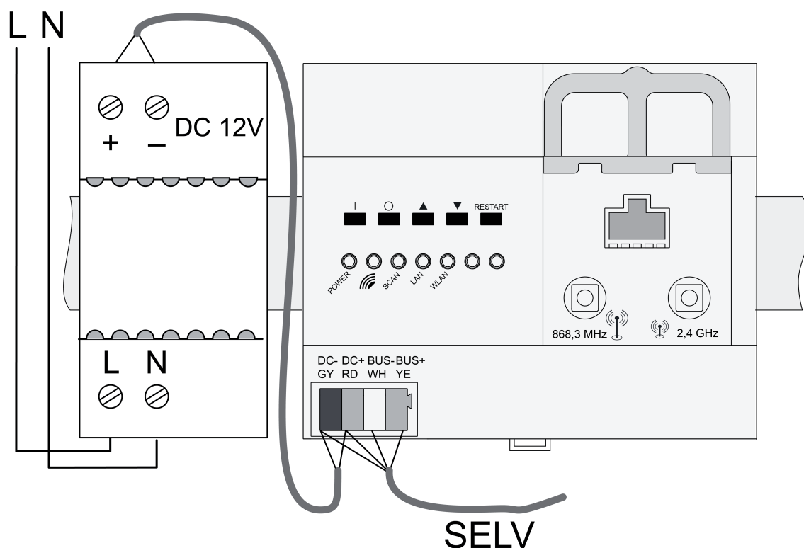
Afbeelding 3: Aansluitschema
