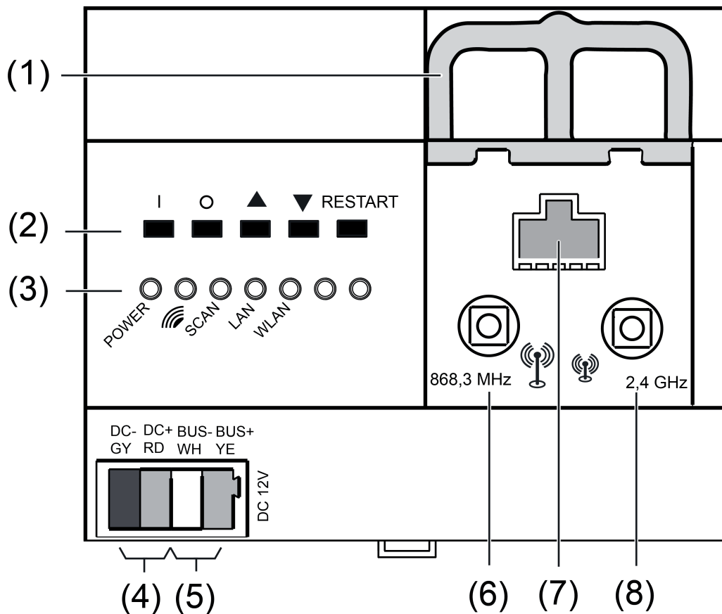
Afbeelding 1: Vooraanzicht eNet-server
