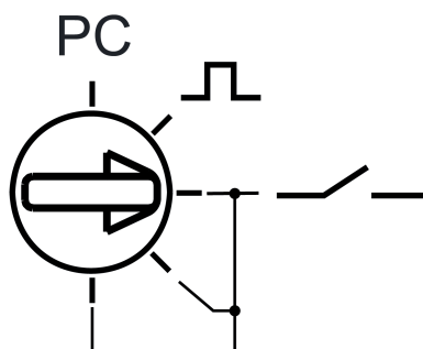
Afbeelding 5: Bedrijfsstandenschakelaar
