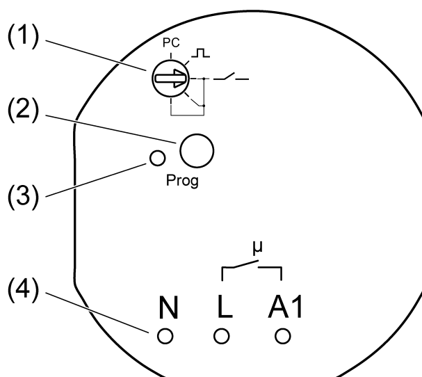
Afbeelding 1: Radiografische schakel-/pulsactor
