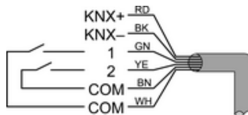
Afbeelding 2: Aansluitbezetting stuurkabel
